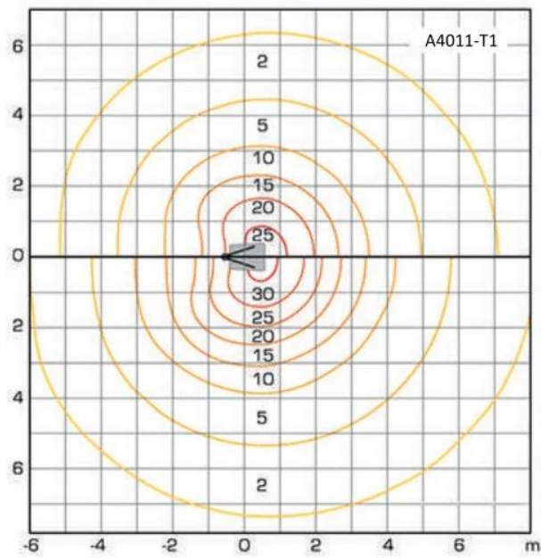
Diagrama dispersia luminii pentru modelul cu 1 brat 70 W / 8400 lm
