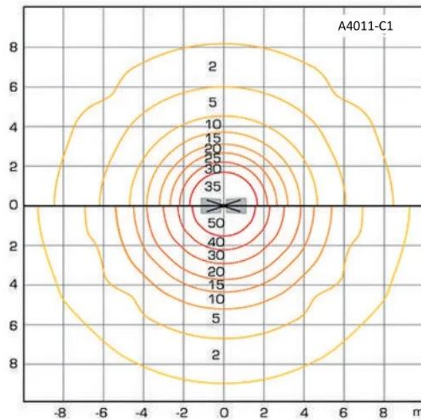
Diagrama dispersia luminii pentru modelul cu 2 brate 140 W / 16800 lm
